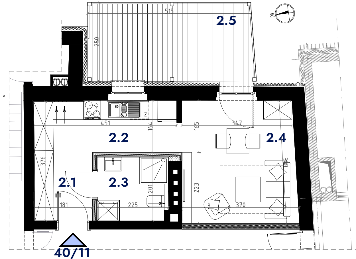
BUDYNEK NR 40 II PIĘTRO
