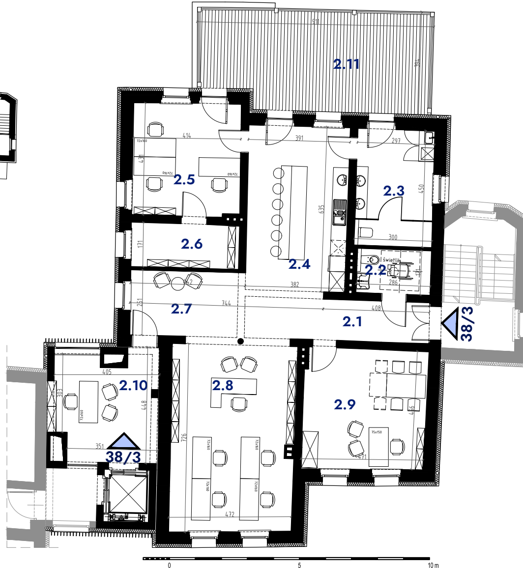
II PIĘTRO
